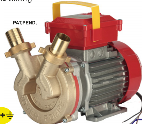
BE-T 40
