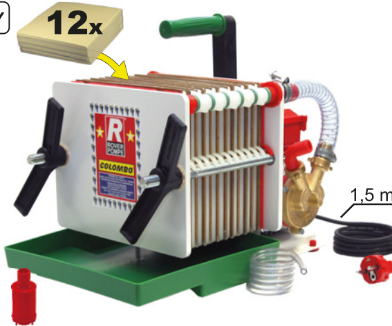
COLOMBO® - 12
